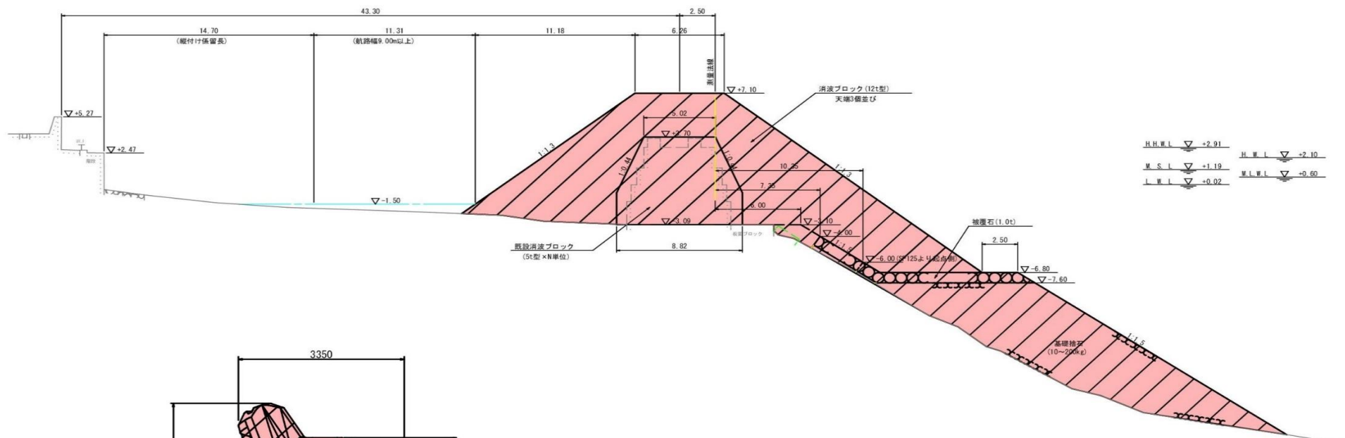
標準断面図
