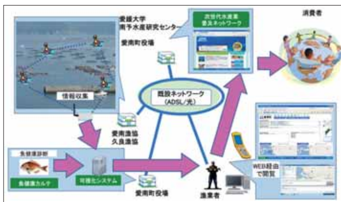
愛南町次世代型水産業振興ネットワークシステム・イメージ詳細図
